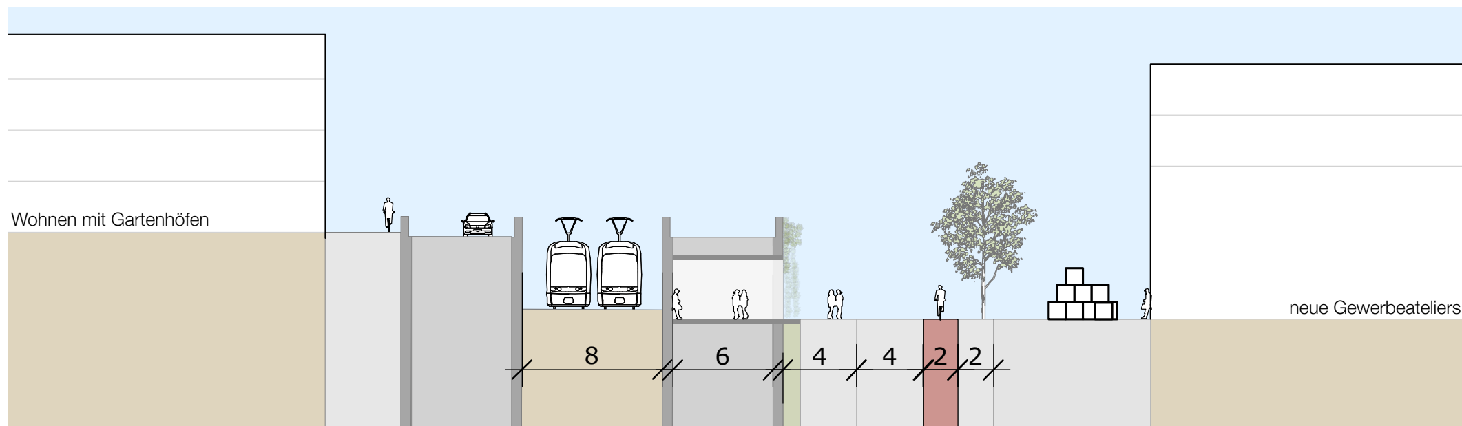
QUERSCHNITT
